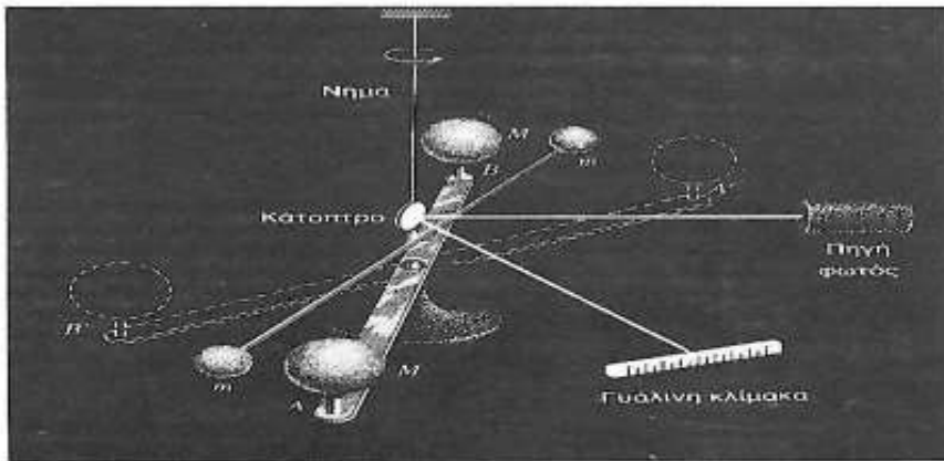
Σχ. 16-4 'Ο ζυγός του Cavendish, που χρησιμοποιείται για την πειραματική επιβεβαίωση του νόμου της παγκόσμιας έλξης του Newton. Οι μάζες m, m αναγκάζονται από ένα νήμα. Οι μάζες M, M μπορούν να περιστρέφονται πάνω σ' ένα σταθερό στήριγμα. Ένα είδωλο του νήματος της λάμπας ανακλάται στο κατόπτρο που είναι συνδεδεμένο στις m, m πάνω στην κλίμακα και έτσι οποιαδήποτε στροφή των m, m μπορεί να μετρηθεί.
