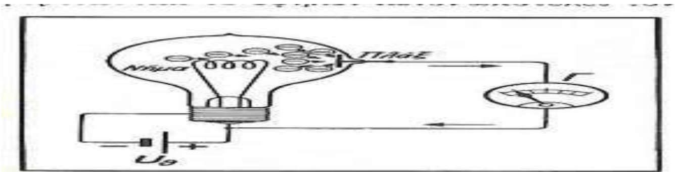
Σχ. 438. "Όταν η πλάτη συνδέεται, μέσω του εὐακισθῆτος γαλβανομέτρου, πρὸς τὸν θετικὸν πόλον πηγῆς συνεχοῦς τάσεως, τὰ ἠλεκτρόνια κινούνται ἐκ τοῦ διαπύρου νήματος πρὸς τὴν πλάτη.
